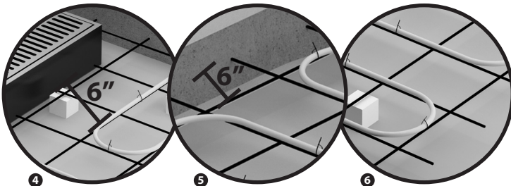
Dégagement des drains et obstacles
