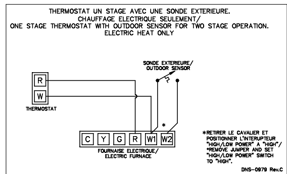
Figure 7: Thermostat 1-stage avec contrôle extérieur pour fonctionnement en mode 2-stages, chauffage électrique seulement
