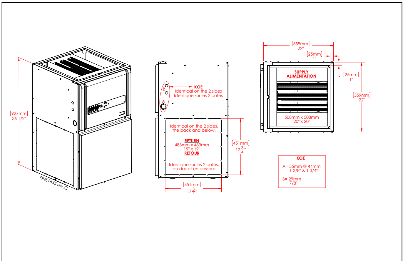
Figure 12: Dimensions modèle Avantage
