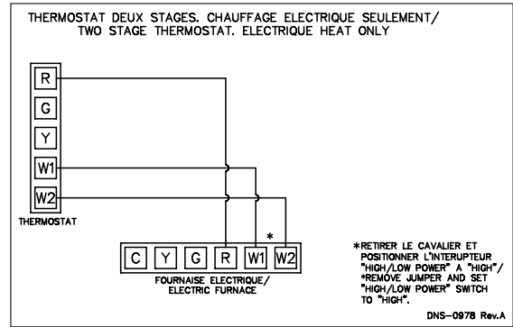
Figure 6: Thermostat 2-stages, chauffage électrique seulement
