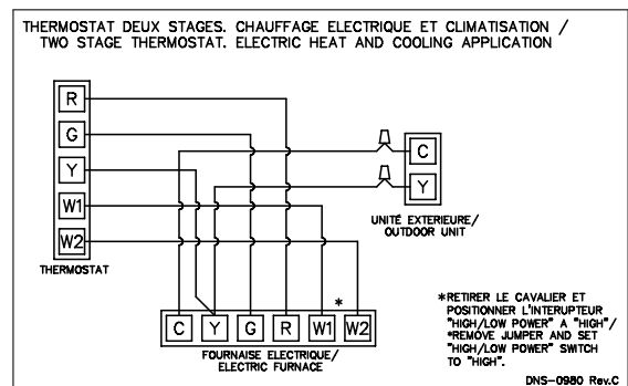
Figure 9: Thermostat 2-stage, chauffage électrique et climatisation
