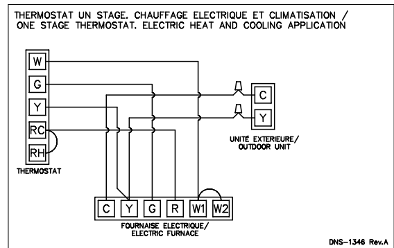
Figure 8: Thermostat 1-stage, chauffage électrique et climatisation
