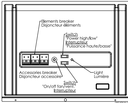
Figure 10: Commandes sur la fournaise Avantage
