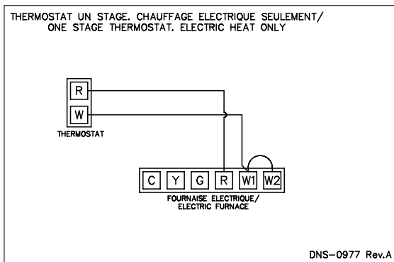
Figure 5: Thermostat 1-stage, chauffage électrique seulement
