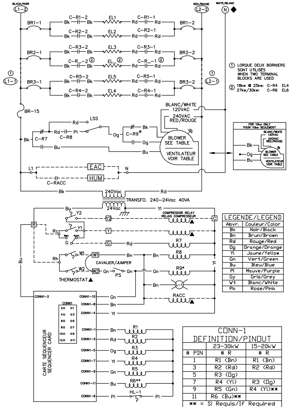
Figure 14: Diagramme électrique, Avantage PSC
