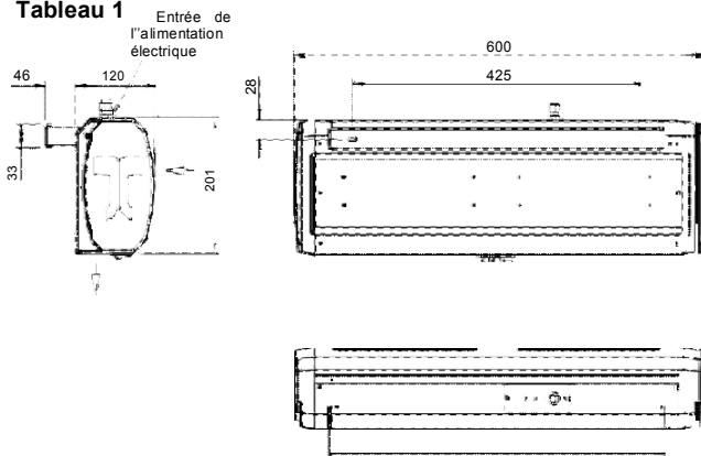
Figure 1 : dessin d'assemblage général du rideau d'air JET 3 HO (LC)
