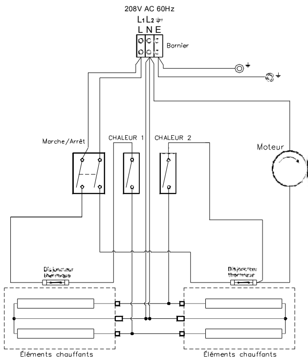
Figure 6 : schéma de câblage du rideau d'air JET 3 HO (LC)
