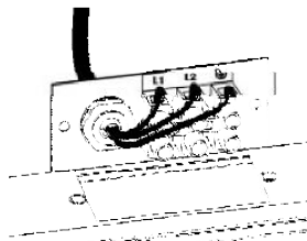
Figure 5 : raccordement électrique
