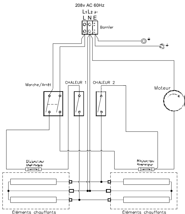
Figure 6 : schéma de câblage du rideau d'air JET 6 (LC)
