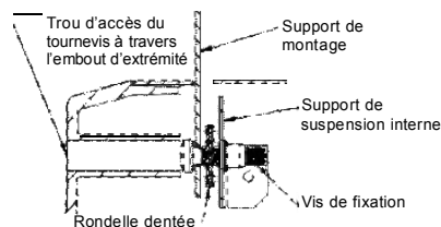
Figure 4 : coupe transversale du support de montage
