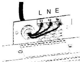
Figure 5 : raccordement électrique
