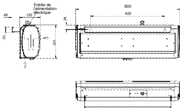
Figure 1 : dessin d'assemblage général du rideau d'air JET 6 (LC)
