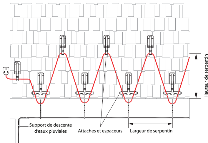
Vue de face du toit
