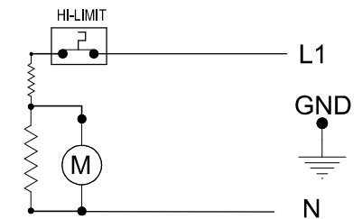
347V Wiring Diagram
