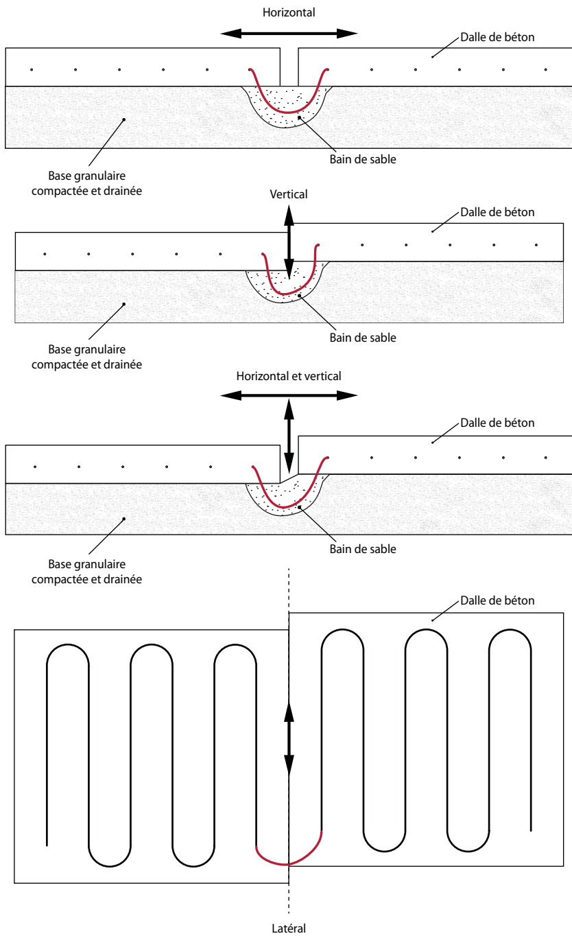
Figure 4 : Mouvements d'un joint d'expansion
